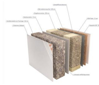
ZENKER Aufbau Außenwand
